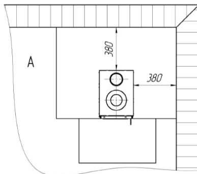
Рисунок 3. Монтаж печи отопительной Kennet Дюймовочка 50
